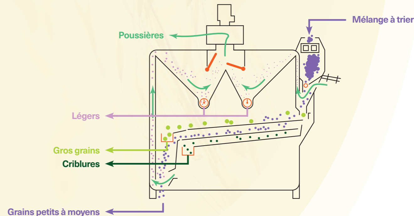
Figure 19 • Schéma légendé du trieur SVD 100
