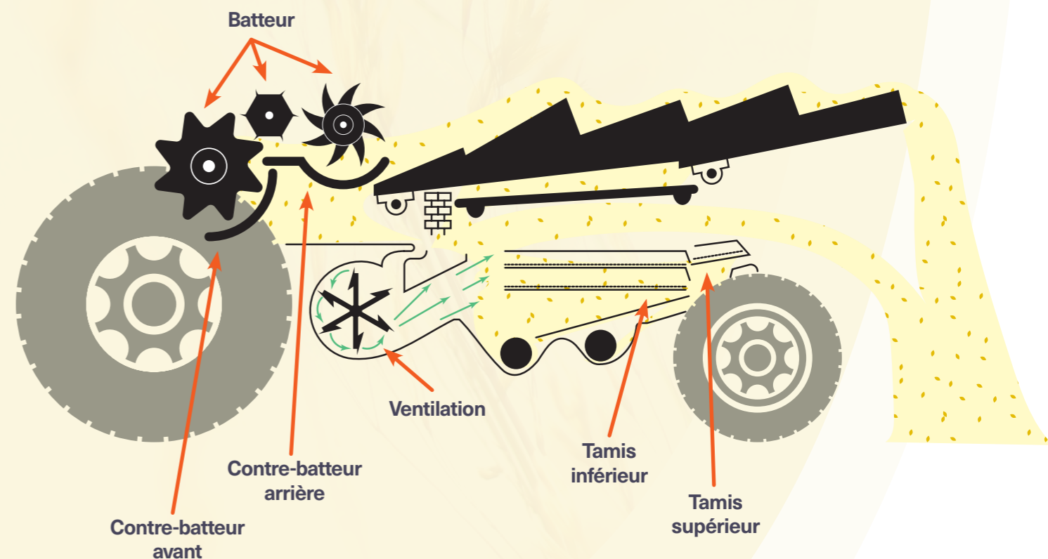
Figure 17 • Schéma de fonctionnement d'une moissonneuse-batteuse (A. Morrison)
